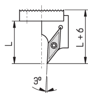
SVUCR11 (Ausführung rechts)
