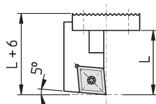
SCLCL09 (Ausführung links)
