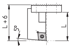
SCLCL06 (Ausführung links)
