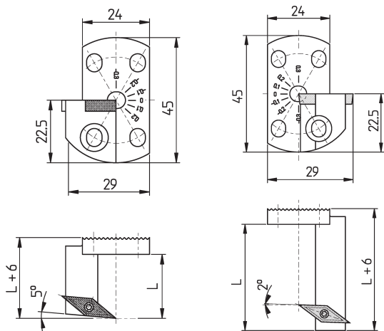
SVJCL11 (Ausführung links)
