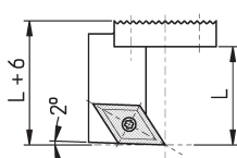
SDJCL11 (Ausführung links)
