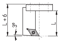
SDJCL07 (Ausführung links)
